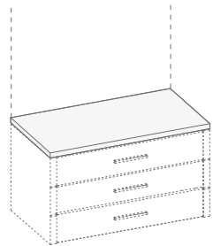
— Top legno sp 30 Wooden top 30
